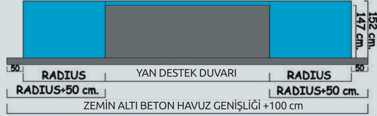
YAN KESİT
