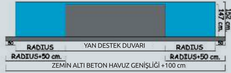
YAN KESİT
